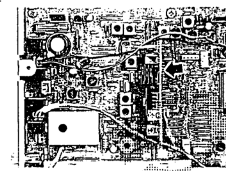
Figure 3 : Installation du module FM
