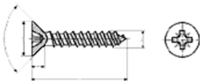
vis-bois-TF-pози-Ragglo.gif
