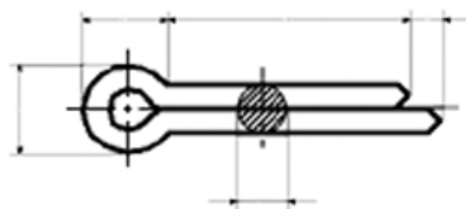
goupille-fendue-R94.gif
