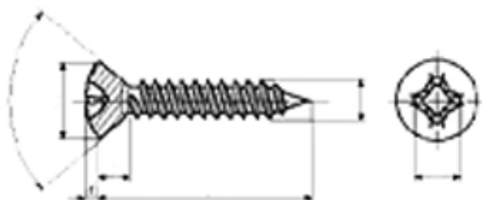
vis-tole-TFB-pozi-R11801.gif
