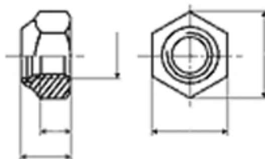
ecrou-securité-bague-nylon-R1722.gif
